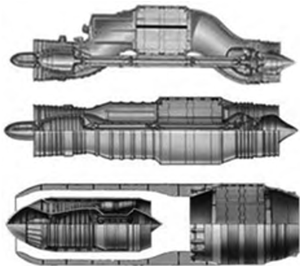
Двигатели атомолета М-60
