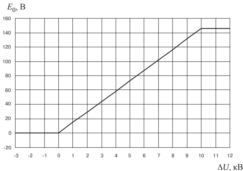
Рис. 5.1. Пример регулировочной характеристики
