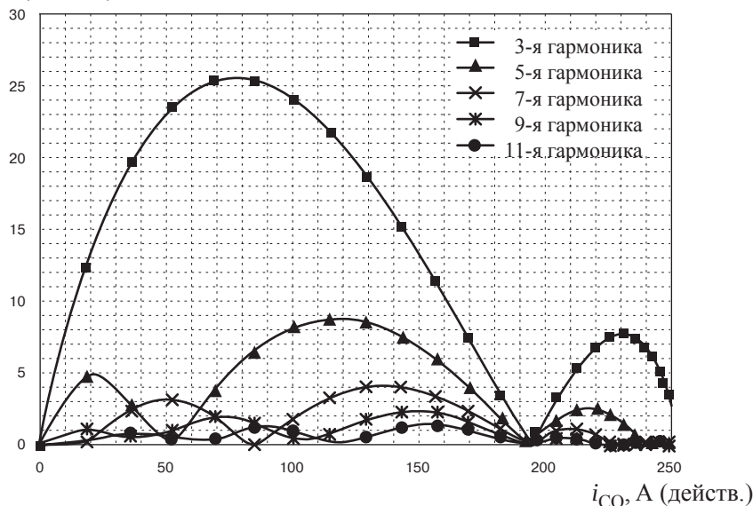
Рис. 3.12. Зависимость величины гармонических составляющих от тока сетевой обмотки реактора (номинальный ток реактора 200А). Компенсационная обмотка отсутствует
