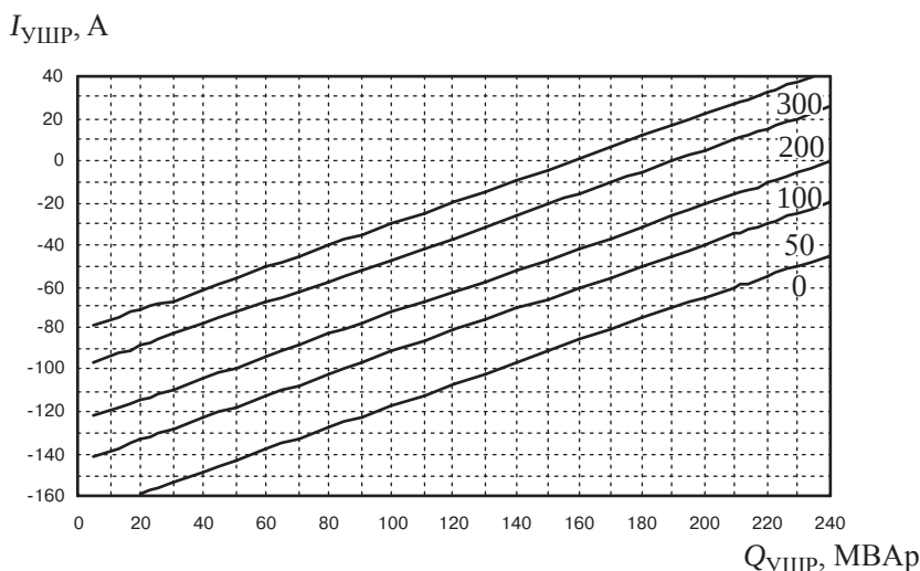
Рис. 7.4. Подпитка дуги от УШР 500 кВ (расчет по (7.3а)). Сопротивление 4-го луча варьируется в диапазоне от 0 до 300 Ом
