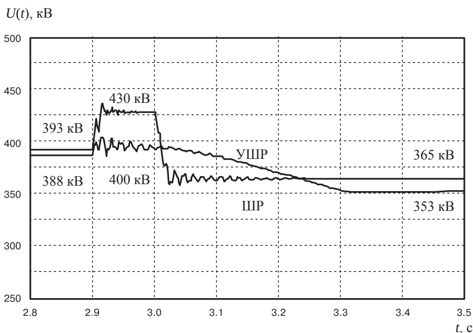
Рис. 6.6. Действующее значение фазного напряжения в схеме рис. 6.2
