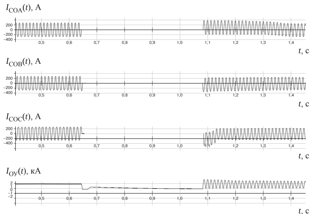
Рис. 11.9. Токи фаз СО и ОУ УШР при имитации цикла ТАПВ на ВЛ 500 кВ
