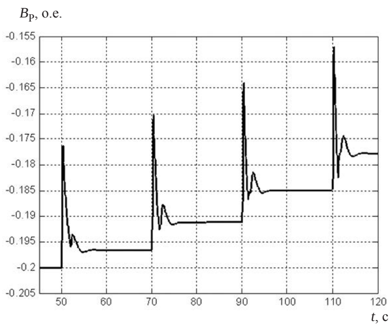
Рис. 2.24, в. Изменение проводимости УШР
