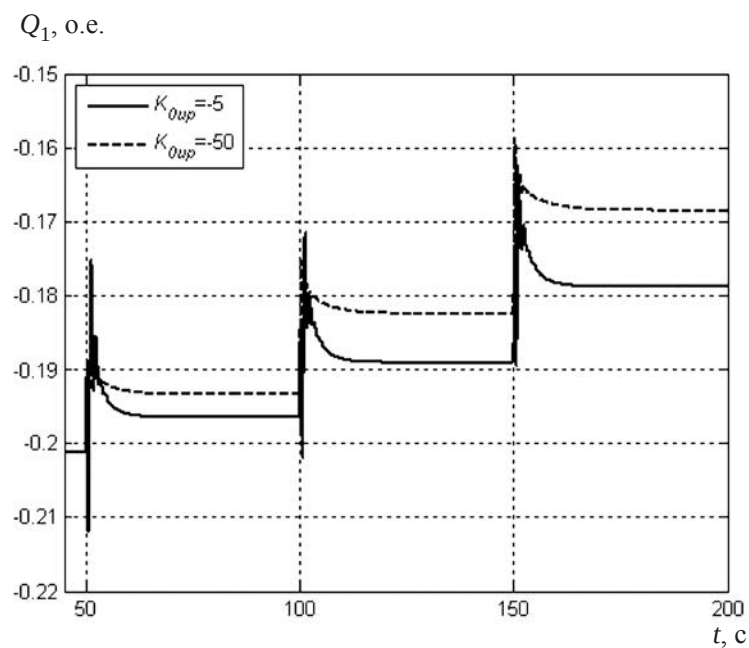
Рис. 2.19, г. Изменение реактивной мощности в начале линии. K_{0u} = -20
