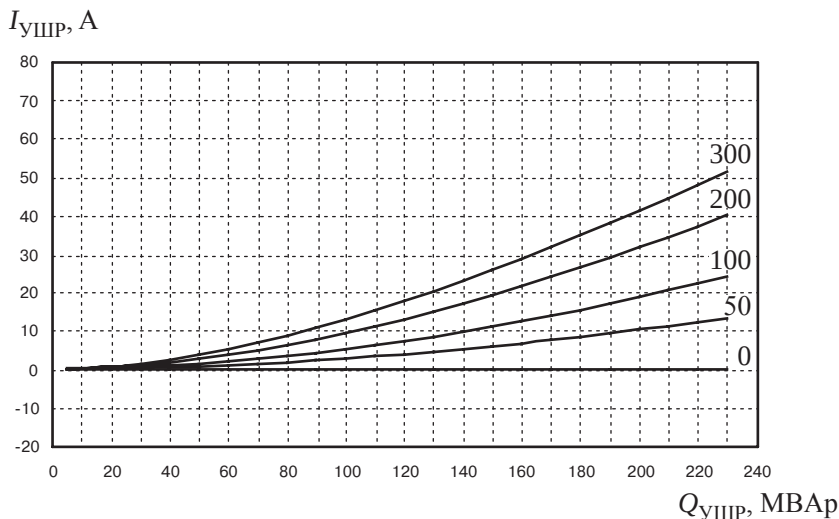
Рис. 7.5. Подпитка дуги от УШР 500 кВ при размыкании треугольника (расчет по (7.36)). Сопротивление 4-го луча варьируется в диапазоне от 0 до 300 Ом
