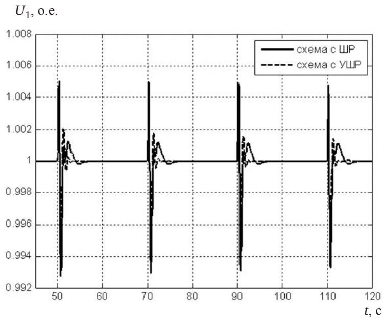
Рис. 2.23, б. Изменение напряжения в точке подключения ШР/УШР (на шинах станции)
