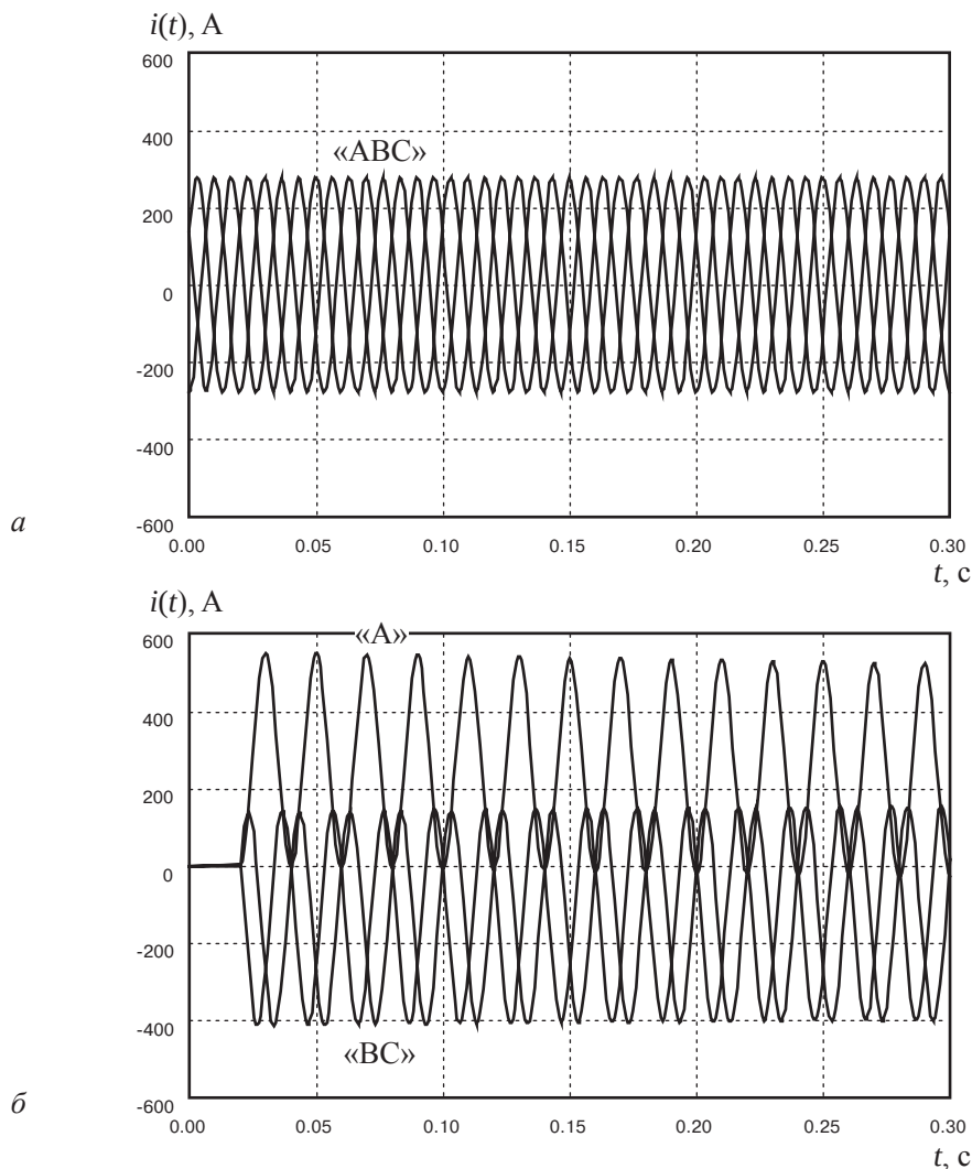
Рис. 8.2. Фазные токи ШР 500 кВ 180 МВАр при его включении в схеме рис. 8.1: а — в установившемся режиме работы; б — в переходном процессе включения реактора в момент времени, когда мгновенное значение напряжения фазы «А» сети имеет нулевое значение
