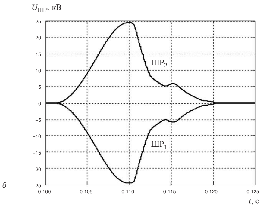
Рис. 10.7. Напряжение на выводах ОУ при включении УШР в моменты прохождения напряжений фаз через ноль ( а ) и падения напряжения на шунтирующих резисторах ( б )
