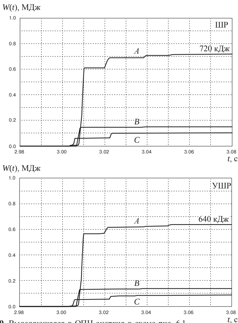
Рис. 6.9. Выделяющаяся в ОПН энергия в схеме рис. 6.1
