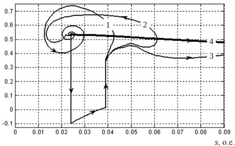
Рис. 9.10. Изменение электромагнитного и тормозного моментов асинхронного электродвигателя при различном быстродействии УПР: 1 — электромагнитный момент асинхронного электродвигателя при \tau_p = 0,3 с; 2 — электромагнитный момент асинхронного электродвигателя при \tau_p = 3,0 с; 3 — электромагнитный момент асинхронного электродвигателя при \tau_p = 4,5 с; 4 — тормозной момент асинхронного электродвигателя
