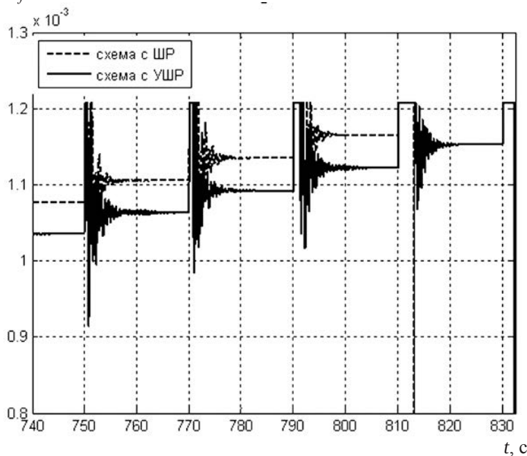
Рис. 2.26, г. Напряжение возбуждения генератора. K_{0u} = -50 , K_{0up} = -15
