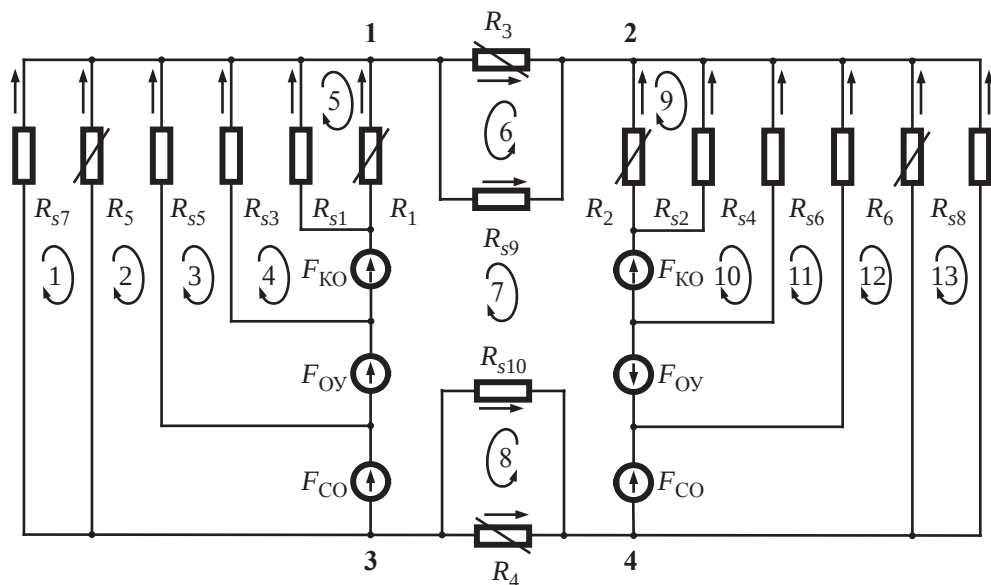
Рис. 4.2. Схема замещения магнитной системы фазы УШР
