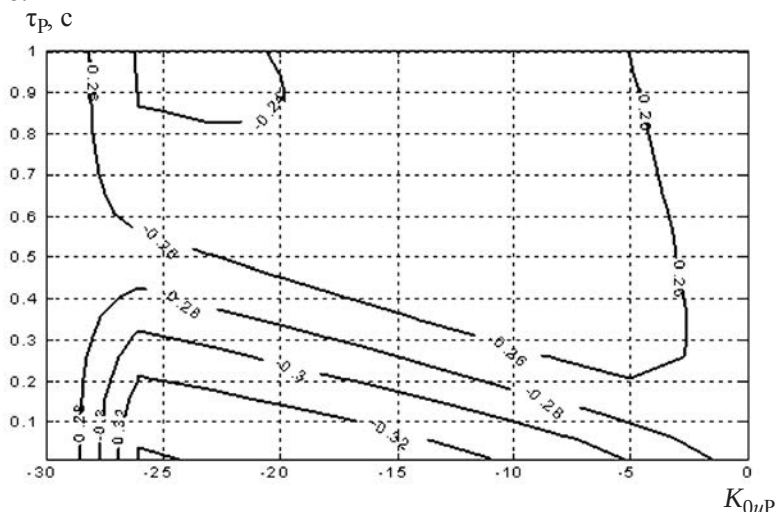
Рис. 2.11. Зависимость показателей колебательной устойчивости от коэффициента усиления канала регулирования по отклонению напряжения и постоянной времени УШР (при K_{0и} = -20 )
