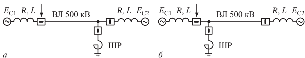
Рис. 8.3. Включение на холостой ход линии с реактором: а — реактор установлен в конце ВЛ; б — реактор установлен в начале ВЛ
