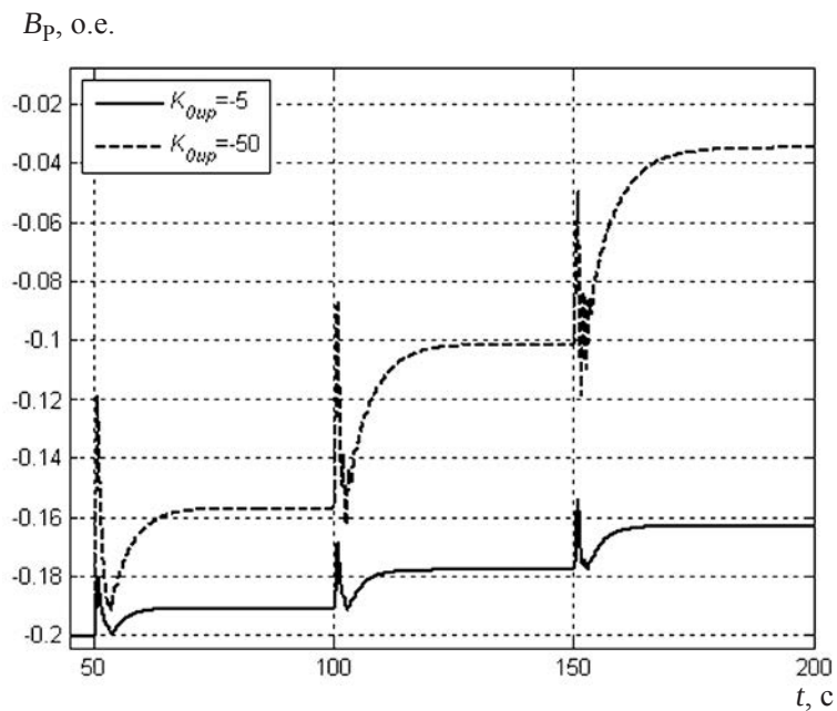
Рис. 2.19, в. Изменение проводимости УШР. K_{0u} = -20
