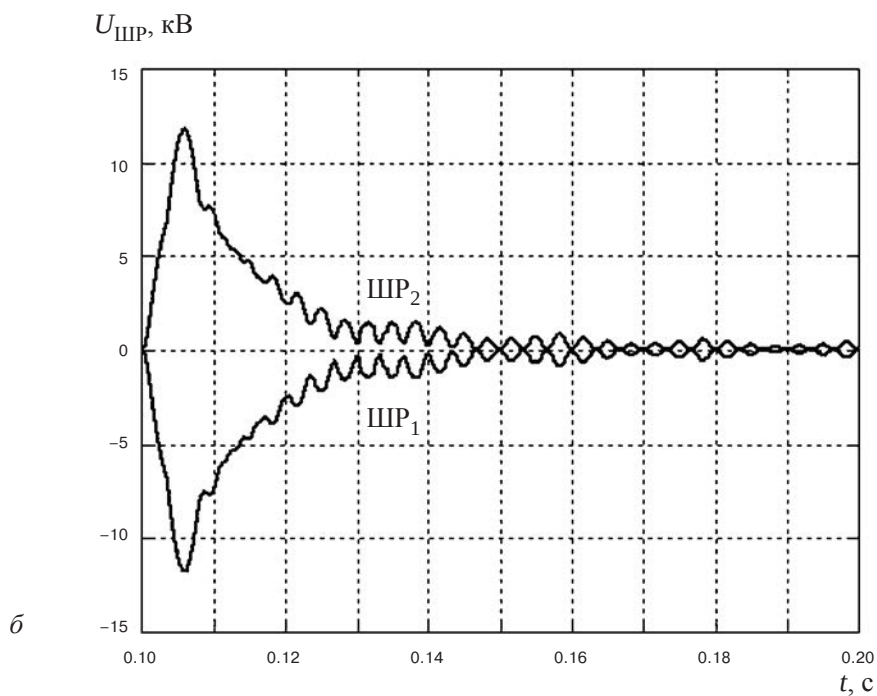
Рис. 10.8. Напряжение на выводах ОУ при включении УШР в моменты прохождения напряжений фаз через максимум ( a ) и падения напряжения на шунтирующих резисторах ( б )
