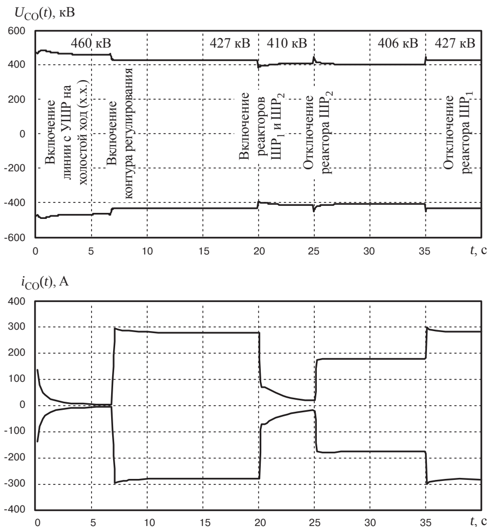
Рис. 5.4. Напряжение и ток СО УШР в схеме рис. 5.3
