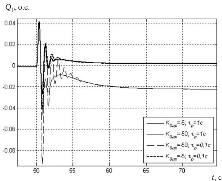
Рис. 2.20, е. Изменение генерируемой реактивной мощности с увеличенной разверткой по времени для t = 50-70 с. K_{Ou} = -50
