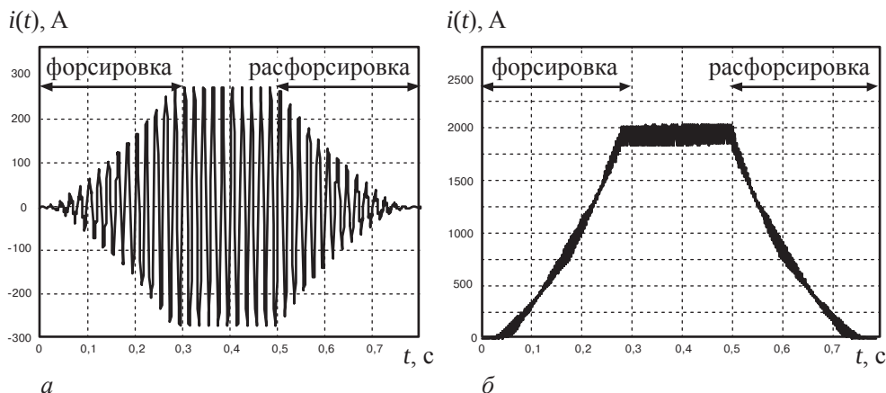
Рис. 3.16. Токи в сетевой обмотке и обмотке управления при форсировке и расфорсировке мощности УШР: а — ток в сетевой обмотке УШР; б — ток в обмотке управления УШР
