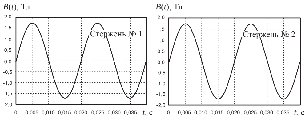
Рис. 3.5. Магнитные индукции в каждом из полустержней (стержни 1, 2) фазы УШР при приложении синусоидального напряжения к сетевой обмотке
