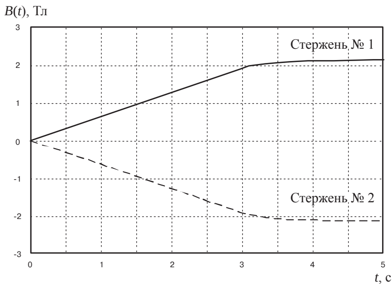
Рис. 3.8. Рост магнитных индукций в каждом из полустержней (стержни 1, 2) фазы УШР при применении номинального постоянного напряжения к обмотке управления
