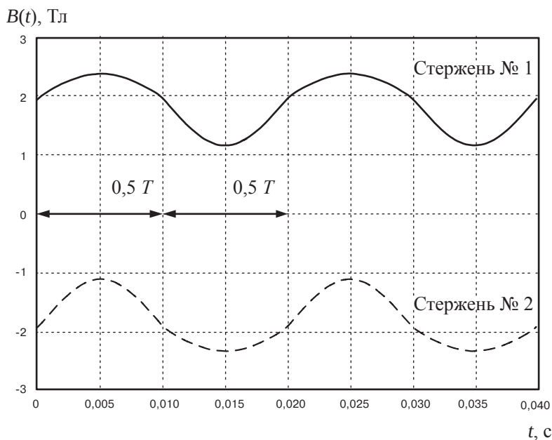
Рис. 3.9. Сложение магнитных потоков (индукций), создаваемых сетевой обмоткой и обмоткой управления, в полустержнях (стержни 1, 2) в номинальном режиме
