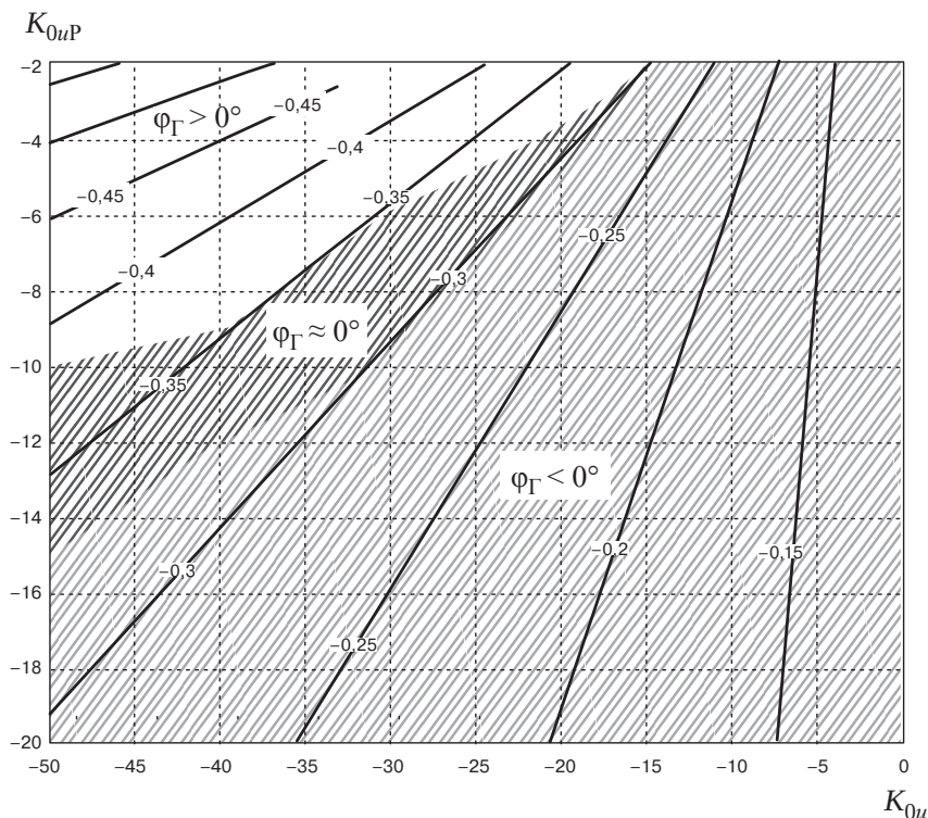
Рис. 2.21. Координация настроек регуляторов генератора K_{0u} и УШР K_{0uP} для обеспечения заданного режима генератора по реактивной мощности (зоны разного оттенка (цвета), определяемых с помощью кривых равного затухания основной составляющей апериодической движения)
