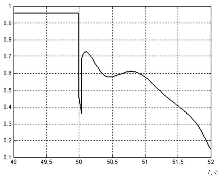
Рис. 9.4. Изменение напряжения в узле нагрузки потребителя
