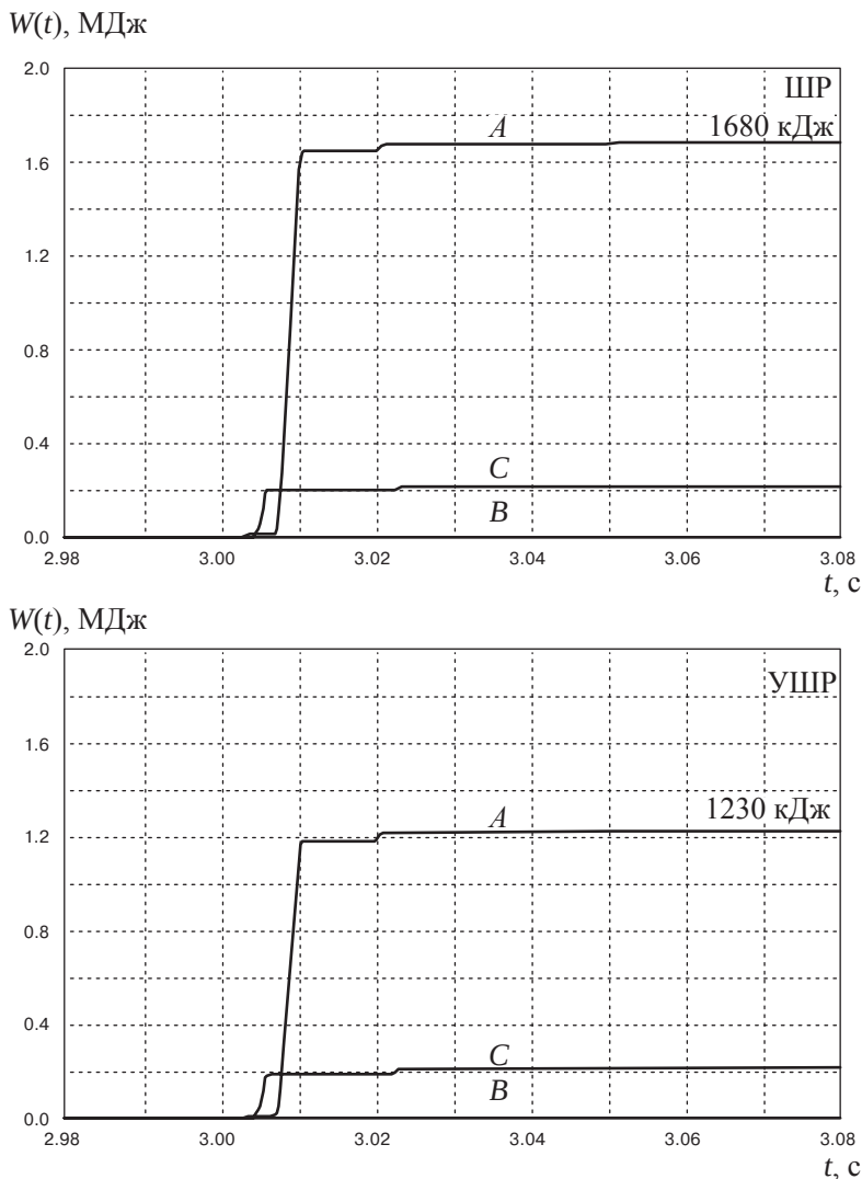
Рис. 6.11. Выделяющаяся в ОПН энергия в схеме рис. 6.2
