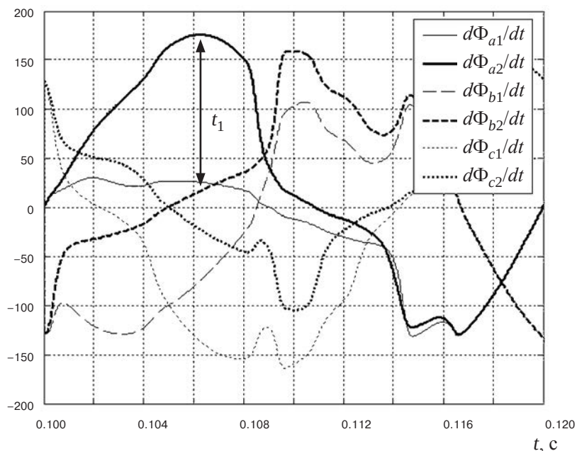
Рис. 10.5, в. Производные потоков полустержней различных фаз при включении УШР в сеть в ноль напряжения фазы А
