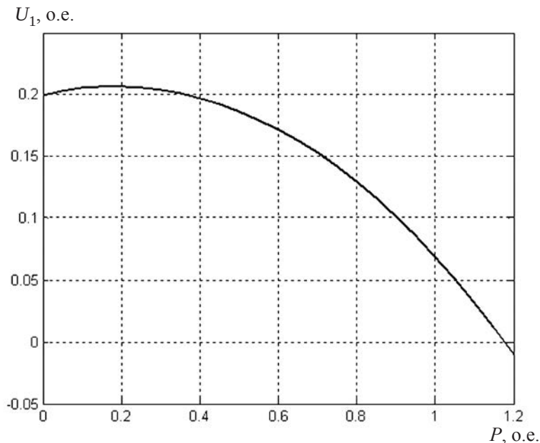
Рис. 2.18. Зависимость необходимой мощности УШР от передаваемой активной мощности для обеспечения режима работы генераторов с \cos \varphi_T = 1
