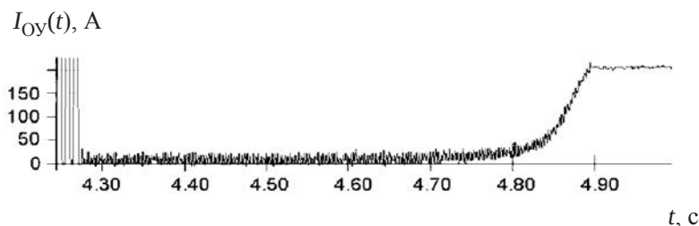
Рис. 11.8. Ускоренное (по сравнению с процессом на рис. 11.7) нарастание тока в режиме предварительного подмагничивания за 0,6 с
