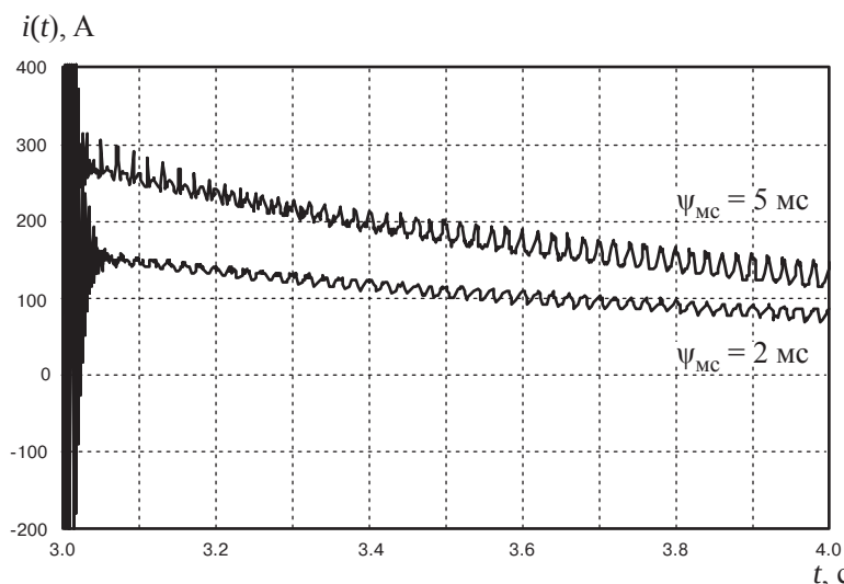
Рис. 8.17. Ток фазы «А» выключателя ВЛ 500 кВ 175 км при ее включении совместно с предварительно подмагниченным УШР 500 кВ 180 МВАр:
