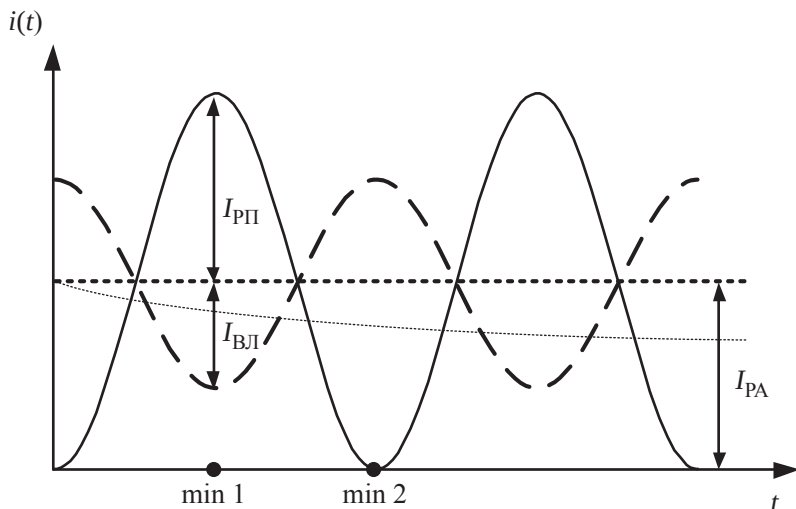
Рис. 8.13. Составляющие тока выключателя ВЛ с шунтирующими реакторами
