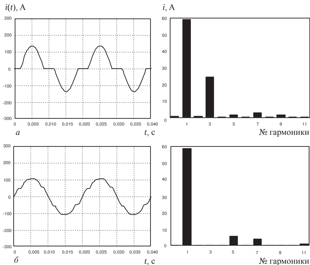
Рис. 3.14. Токи сетевой обмотки и их гармонический состав в режиме потребления 40 % от номинальной мощности УШР: а — КО разомкнута; б — КО замкнута
