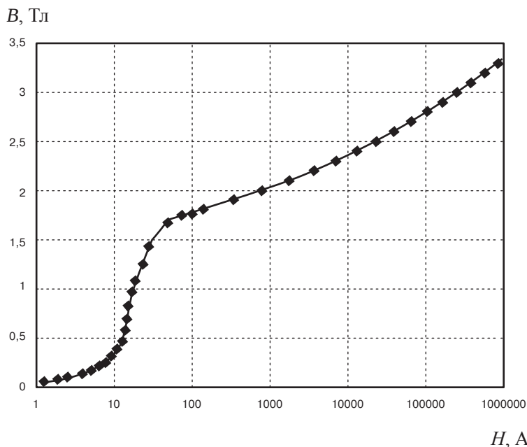
Рис. 4.4. Характеристика намагничивания стали, используемая при моделировании УШР
