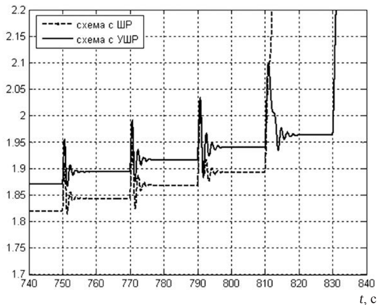
Рис. 2.26, б. Абсолютный угол ротора генератора. K_{0u} = -50 , K_{0uP} = -15
