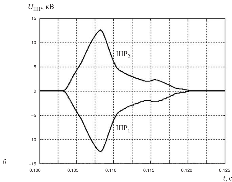
Рис. 10.9. Напряжение на выводах ОУ при включении УШР (а) и падение напряжения на шунтирующих резисторах (б)
