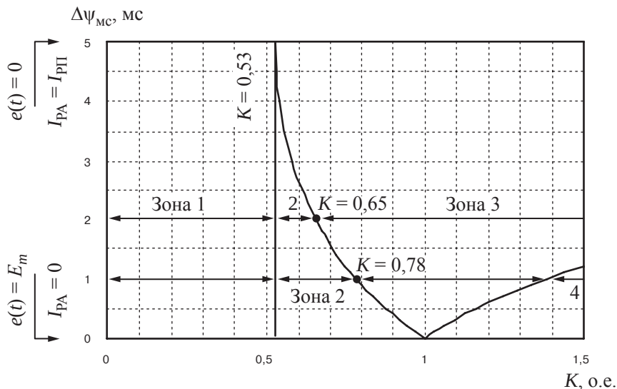
Рис. 8.15. Область применения различных мероприятий для ограничения апериодических токов
