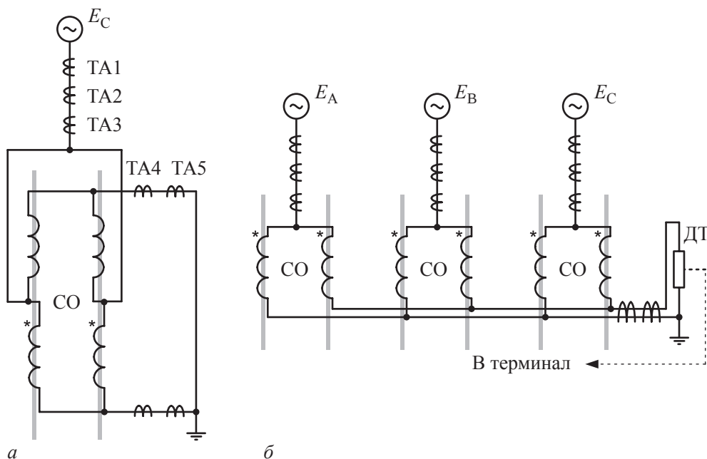
Рис. 11.6. Релейная защита сетевой обмотки: а — размещение встроенных ТТ на отводах нейтралей СО; б — поперечная дифференциальная токовая защита с применением датчика тока (ДТ)
