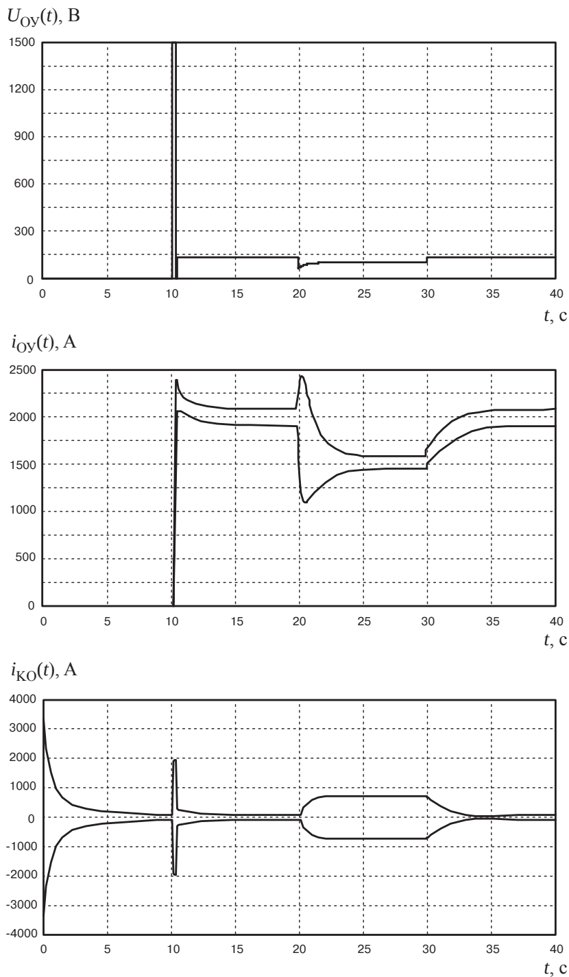
Рис. 5.8. Приложенное к ОУ напряжение, токи ОУ и КО в схеме рис. 5.6
