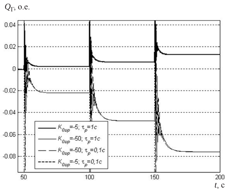
Рис. 2.20, д. Изменение генерируемой реактивной мощности. K_{Ou} = -50
