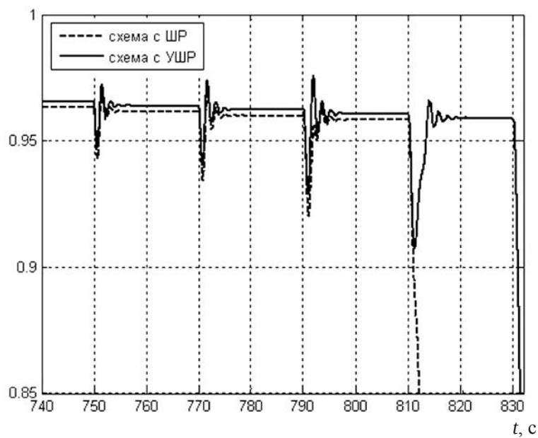
Рис. 2.26, в. Напряжение в точке подключения ШР/УШР (на шинах станции). K_{0u} = -50 , K_{0up} = -15
