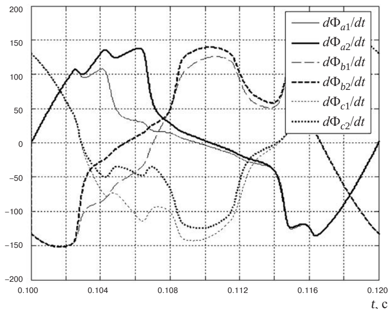
Рис. 10.9, в. Производные потоков полустержней различных фаз при включении УШР в сеть
