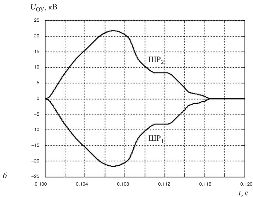
Рис. 10.5. Напряжение на выводах ОУ при включении УШР в ноль напряжения фазы А (а) и падение напряжения на шунтирующих резисторах (б)
