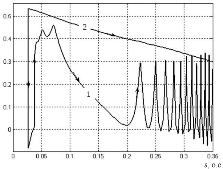
Рис. 9.5. Изменение электромагнитного и тормозного моментов асинхронного электродвигателя: 1 — электромагнитный момент асинхронного электродвигателя; 2 — тормозной момент асинхронного электродвигателя
