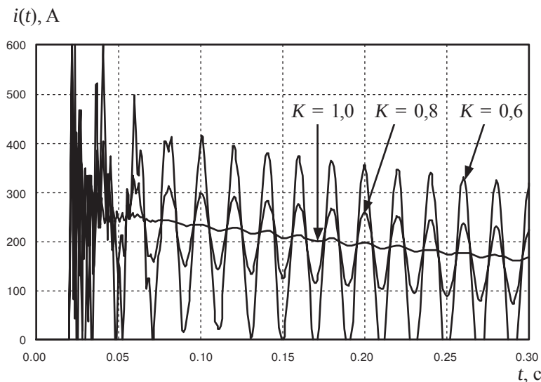
Рис. 8.4. Ток фазы «А» ВЛ 500 кВ различной длины с одним шунтирующим реактором 180 МВАр, установленным на конце ВЛ (схема рис. 8.3, а), при включении линии в момент времени, когда мгновенное значение напряжения фазы «А» равно нулю, в зависимости от длины ВЛ: 175 км ( K \approx 1 ); 220 км ( K = 0,8 ); 290 км ( K = 0,6 )
