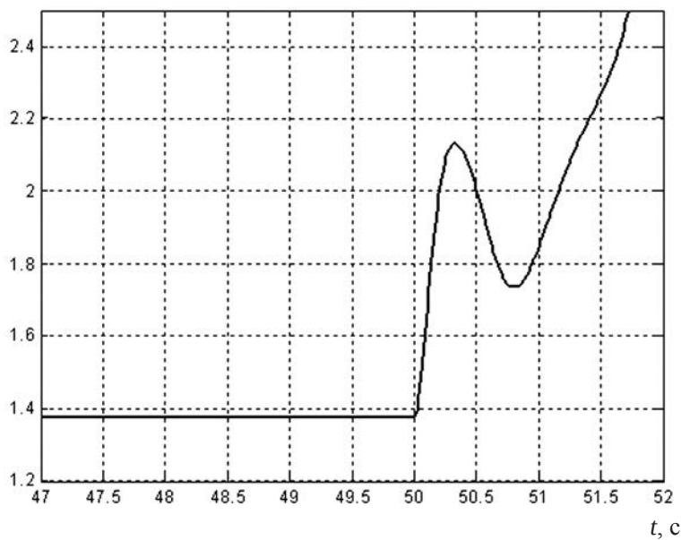
Рис. 9.3. Изменение относительного угла между роторами генератора электрической станции и синхронного электродвигателя
