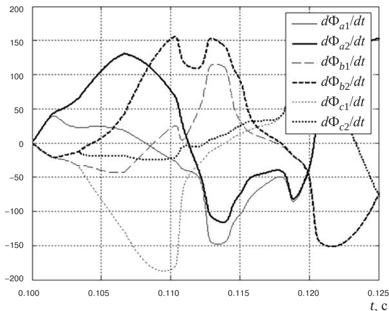
Рис. 10.7, в. Производные потоков полустержней различных фаз при включении УШР в сеть в моменты прохождения напряжений фаз «А», «В», «С» через ноль
