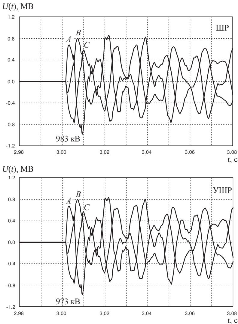
Рис. 6.8. Неограниченные действием ОПН перенапряжения в конце ВЛ в схеме рис. 6.1
