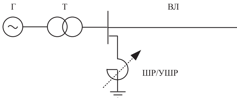
Рис. 2.3. Расчетная схема сети с реактором, установленным на шинах электрической станции
