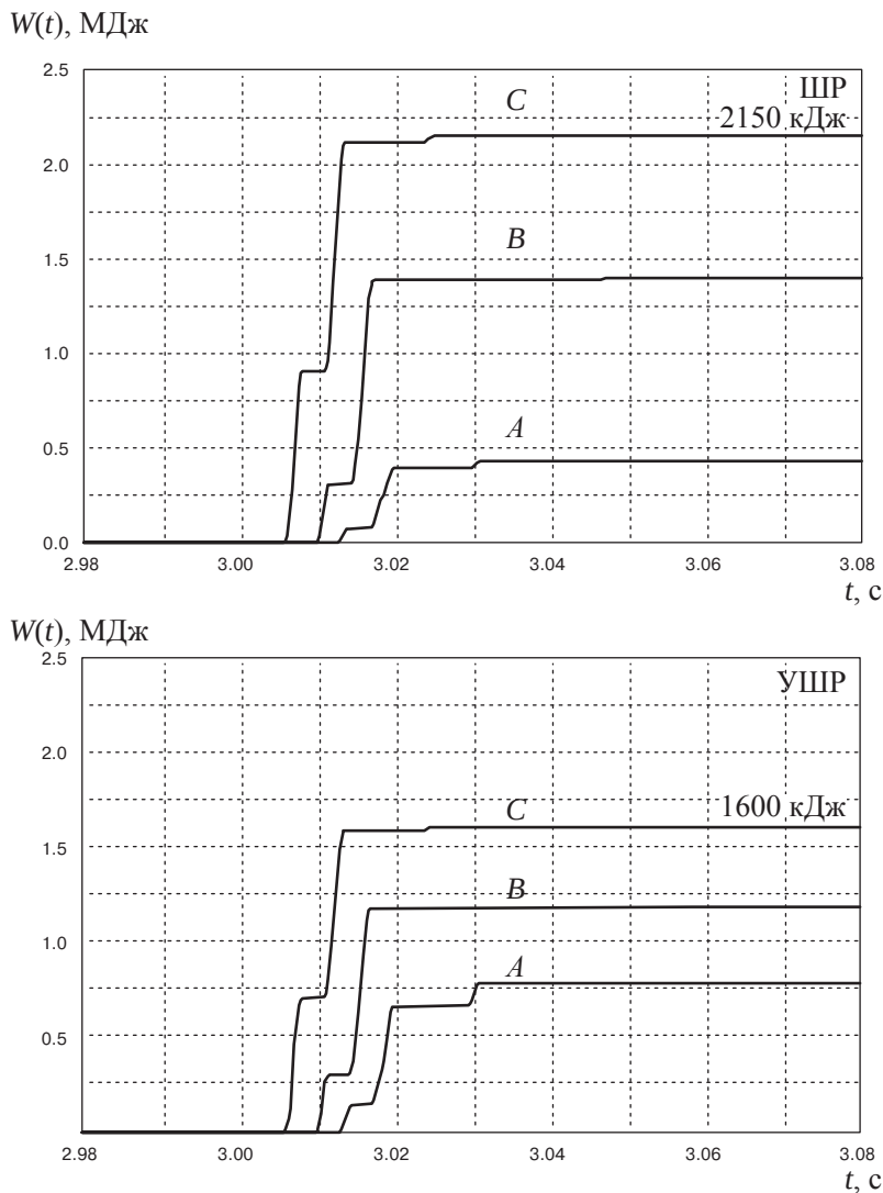
Рис. 6.13. Выделяющаяся в ОПН энергия в схеме рис. 6.3
