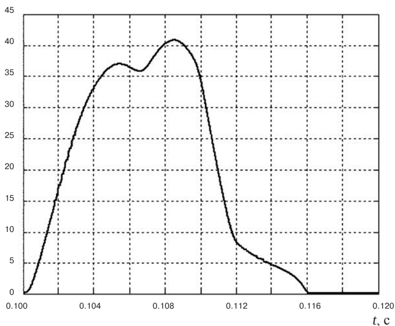
Рис. 10.6, а. Напряжение на выводах ОУ при включении УШР в максимум напряжения фазы А
